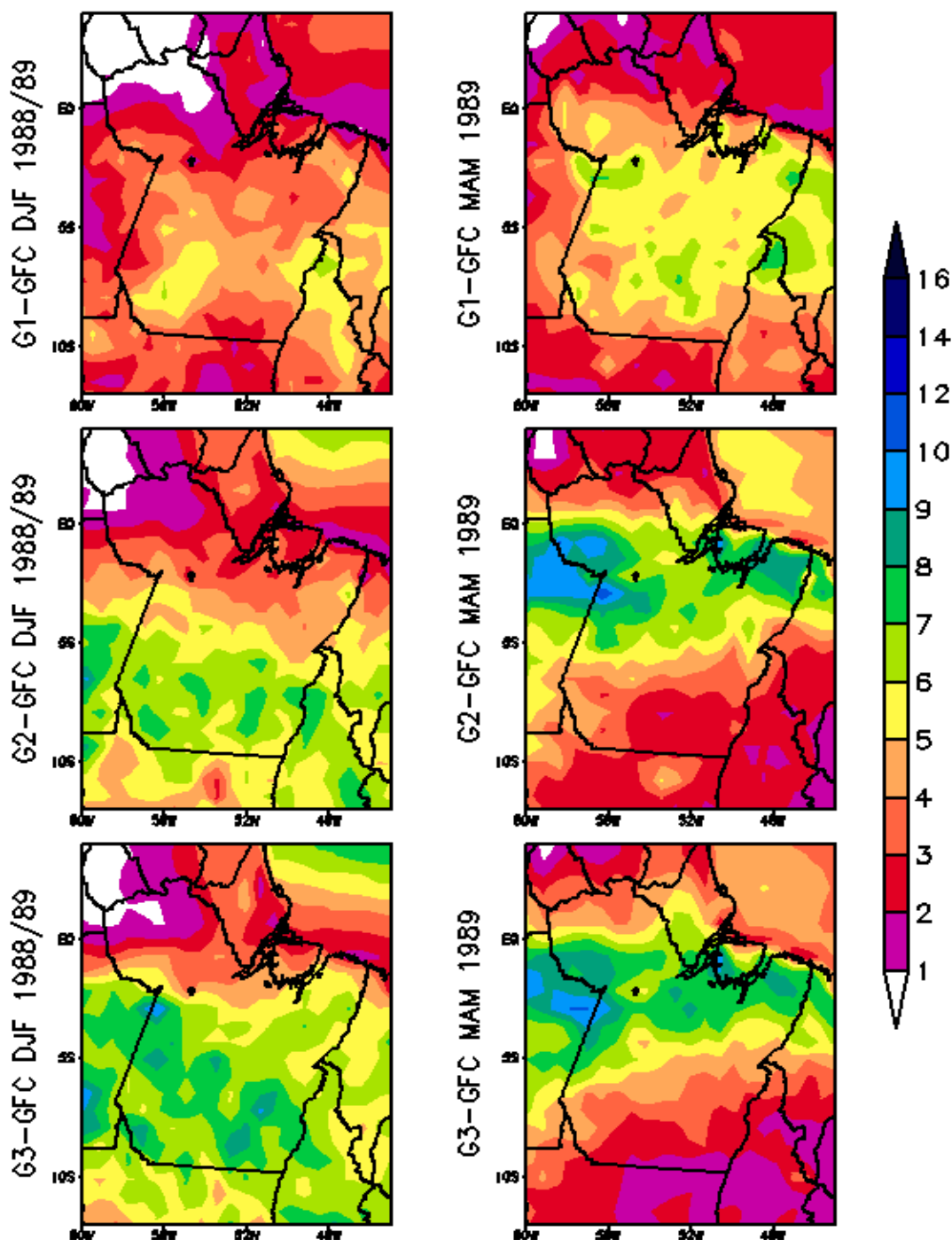
Figura 13. Padrões (distribuição espacial e intensidade) da precipitação (mm/dia) sazonal simulada em DJF 1988/89 e MAM 1989 correspondentes as grades G1 (mapa superior), G2 (mapa intermediário) e G3 (mapa inferior), usando o esquema convectivo GFC.
