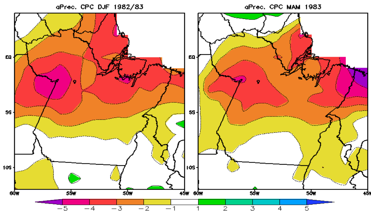
Figura 5. Anomalias de precipitação do CPC observada durante DJF 1982/83 e MAM 1983.
