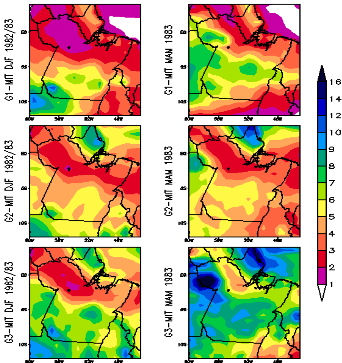
Figura 12. Idem a Figura 11, porém para o esquema convectivo MIT.
