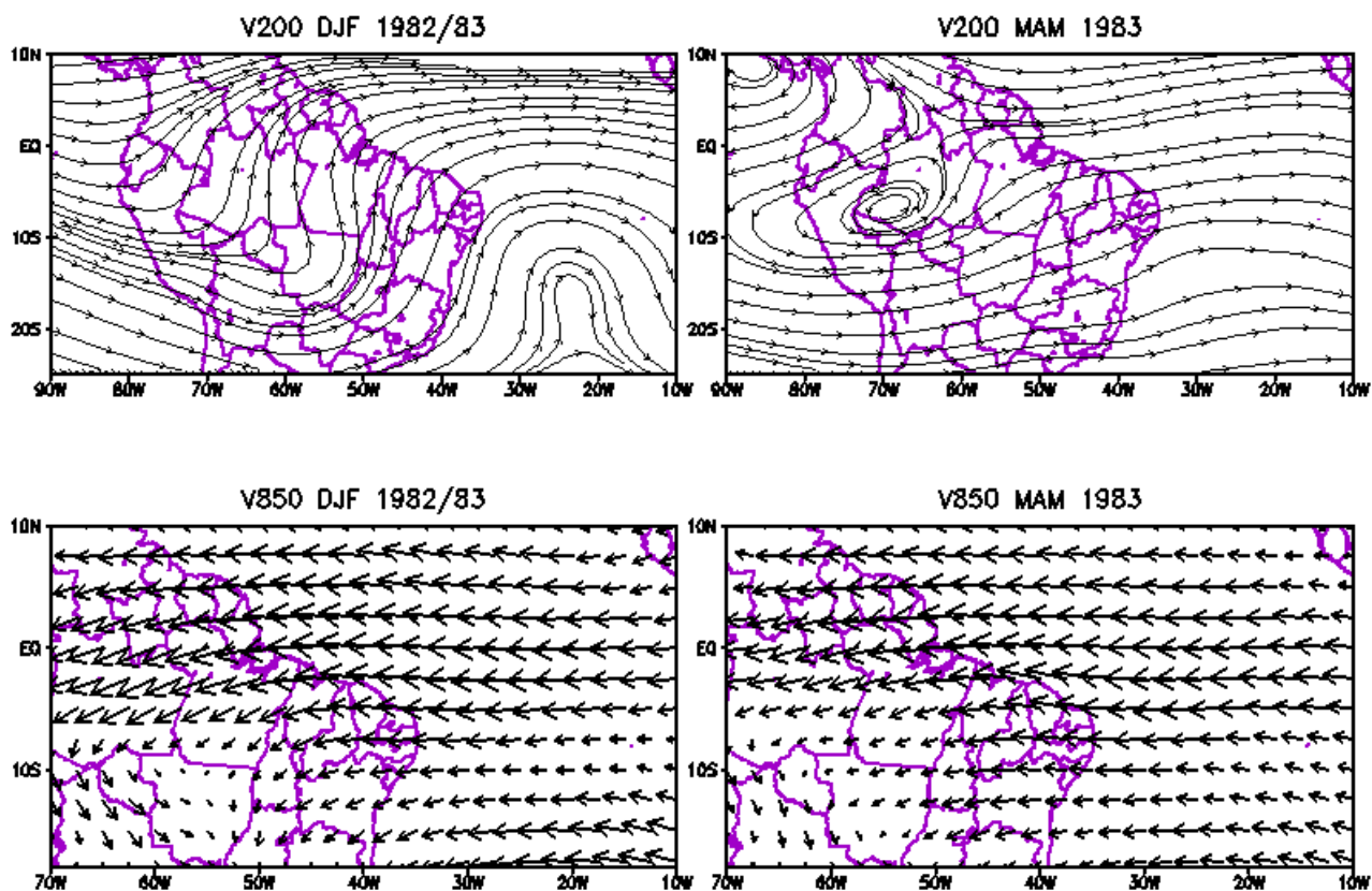
Figura 4. Padrões de vento horizontal em 200 hPa (mapa superior) e em 850 hPa (mapa inferior) durante DJF 1982/83 e MAM 1983.
