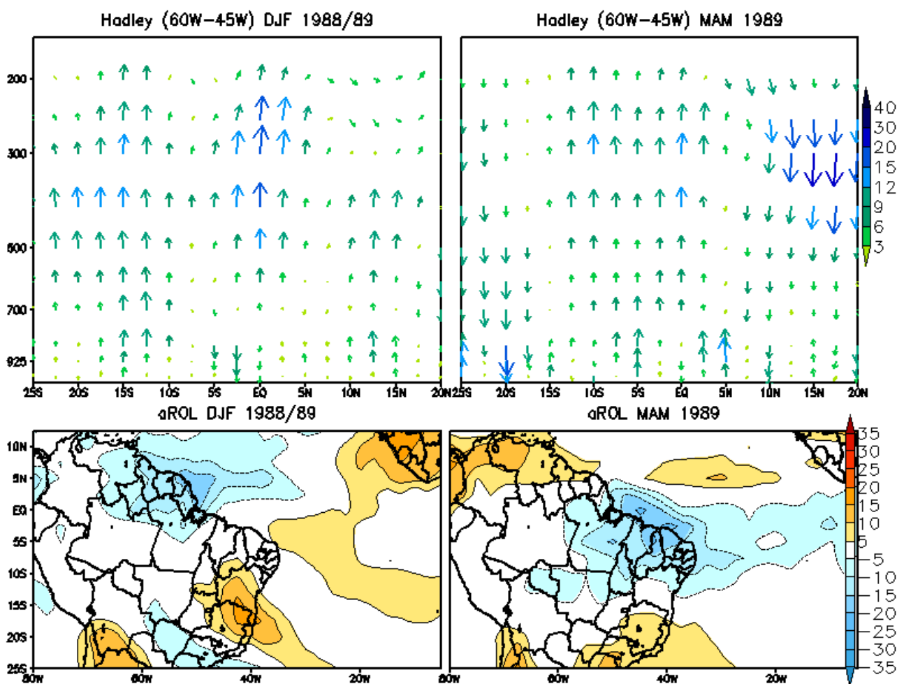
Figura 7. Cortes verticais (latitude x altura) da circulação meridional associada à célula de Hadley média entre 60^{\circ}\text{W}-45^{\circ}\text{W} (mapa superior) e anomalias de ROL (mapa inferior) sobre a América do Sul e Atlântico durante DJF 1988/89 e MAM 1989.
