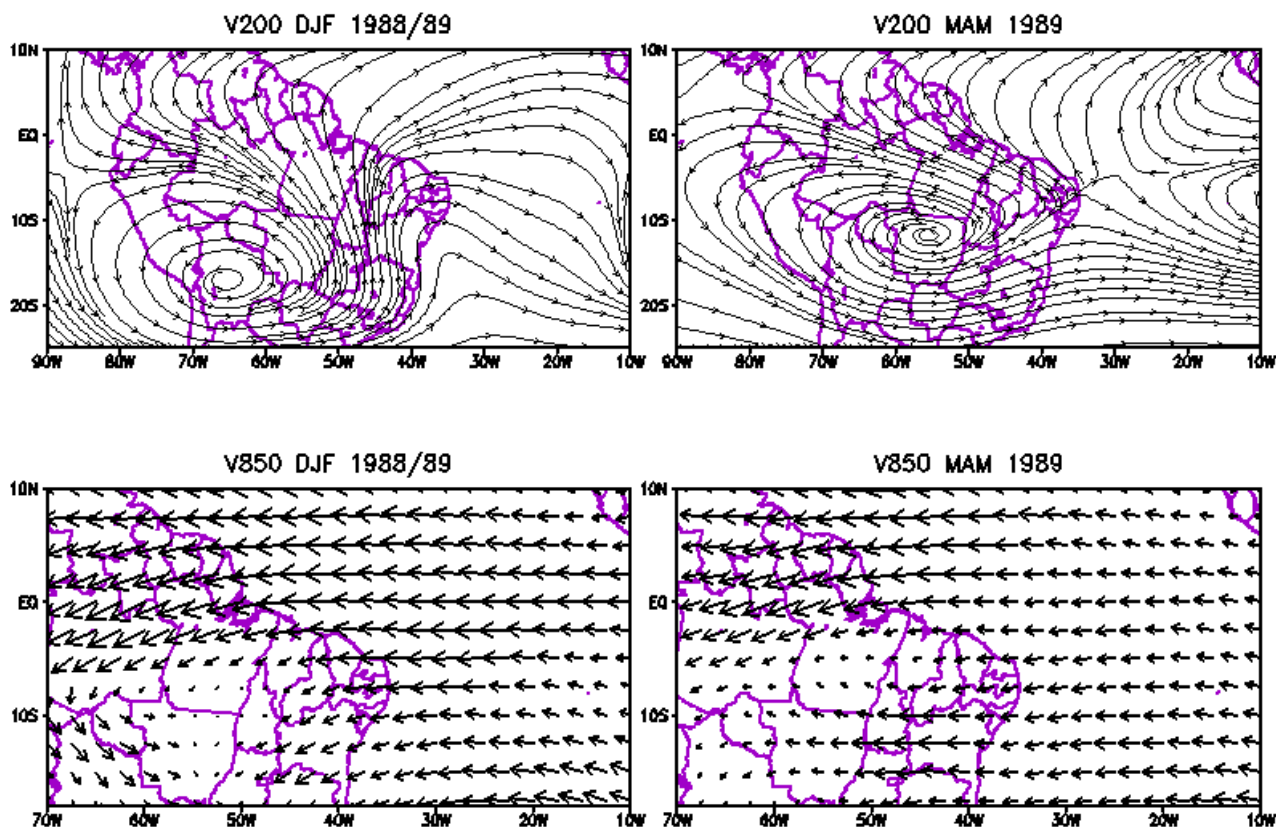
Figura 8. Padrões de vento horizontal em 200 hPa (mapa superior) e em 850 hPa (mapa inferior) durante DJF 1988/89 e MAM 1989.
