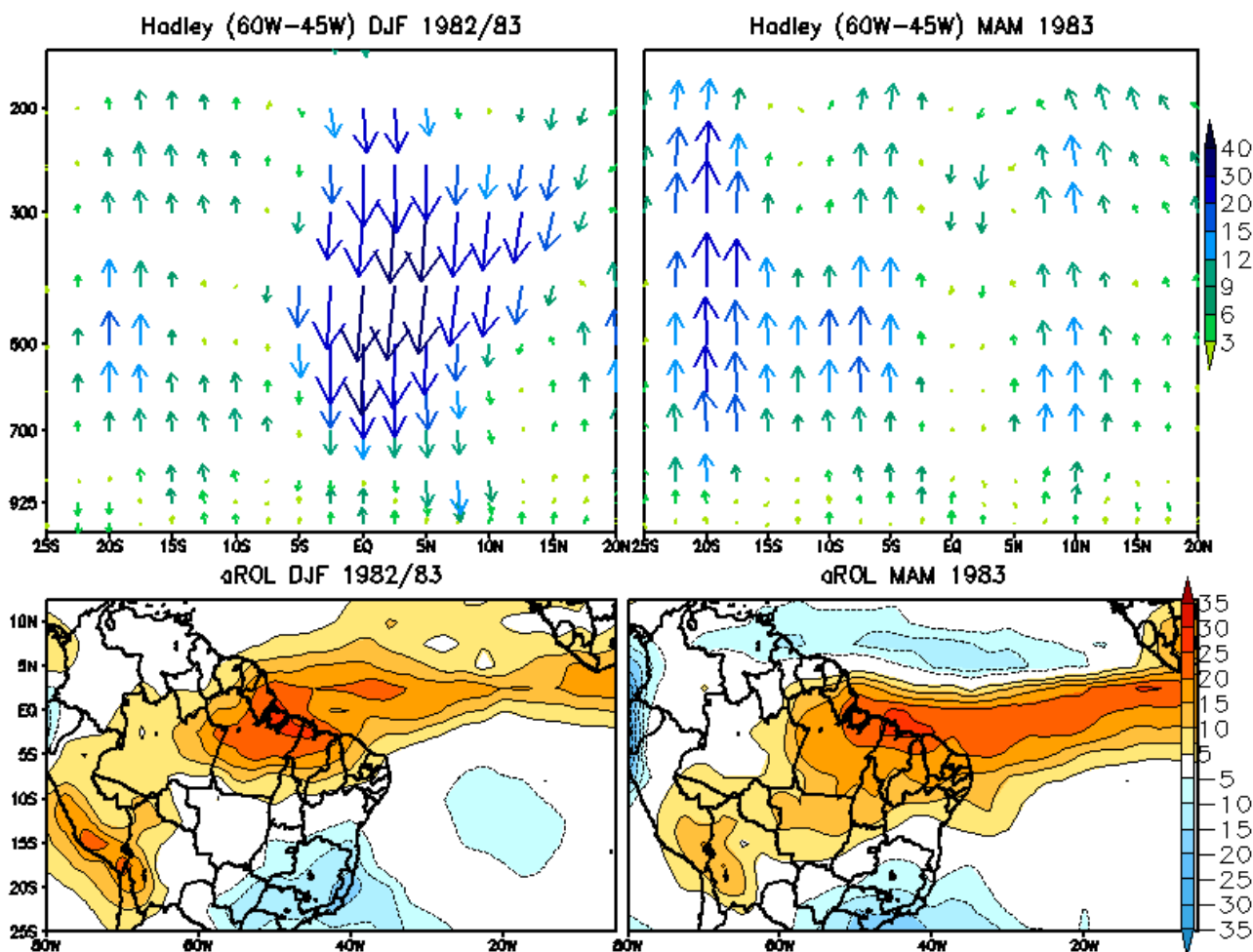
Figura 3. Cortes verticais (latitude x altura) da circulação meridional associada à célula de Hadley média entre 60°W-45°W (mapa superior) e anomalias de ROL (mapa inferior) sobre a América do Sul e Atlântico durante DJF 1982/83 e MAM 1983.
