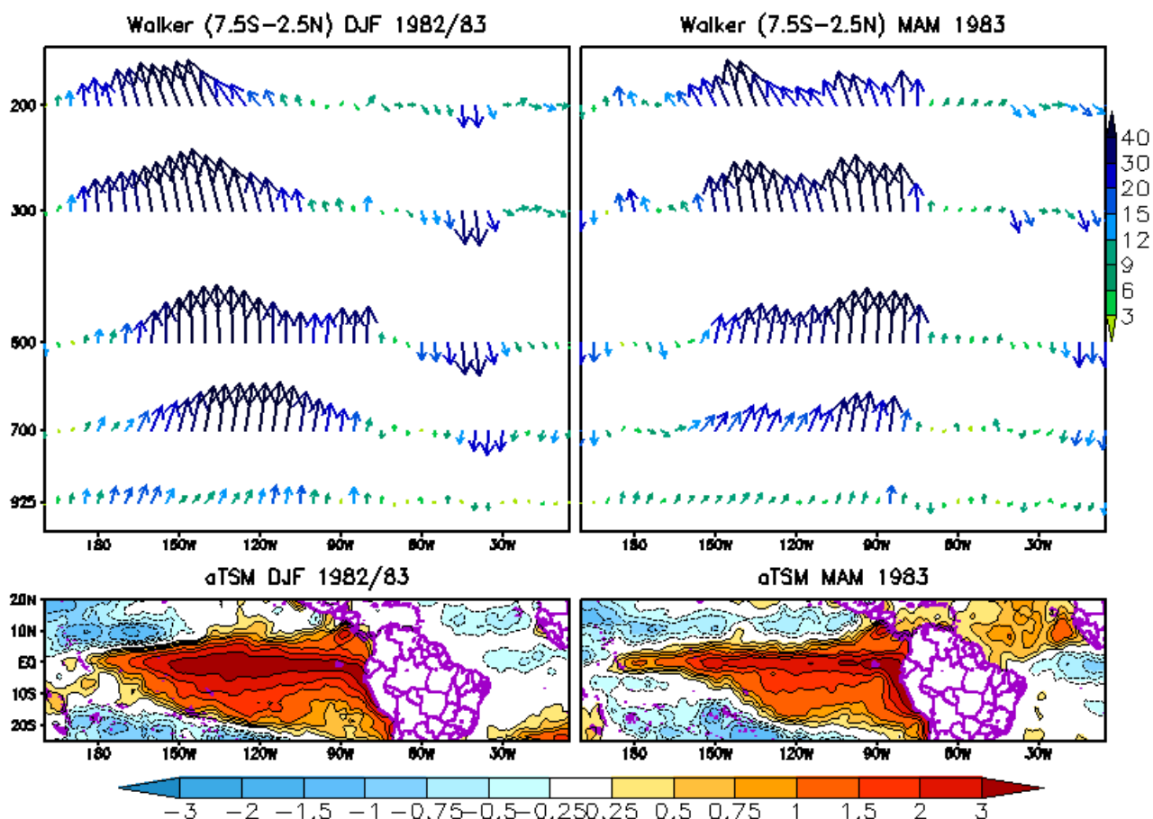
Figura 2. Cortes verticais (longitude x altura) da circulação zonal associada à célula de Walker média entre 7.5°S-2.5°N (mapa superior) e anomalias de TSM (mapa inferior) sobre o Pacífico e Atlântico durante DJF 1982/83 e MAM 1983.
