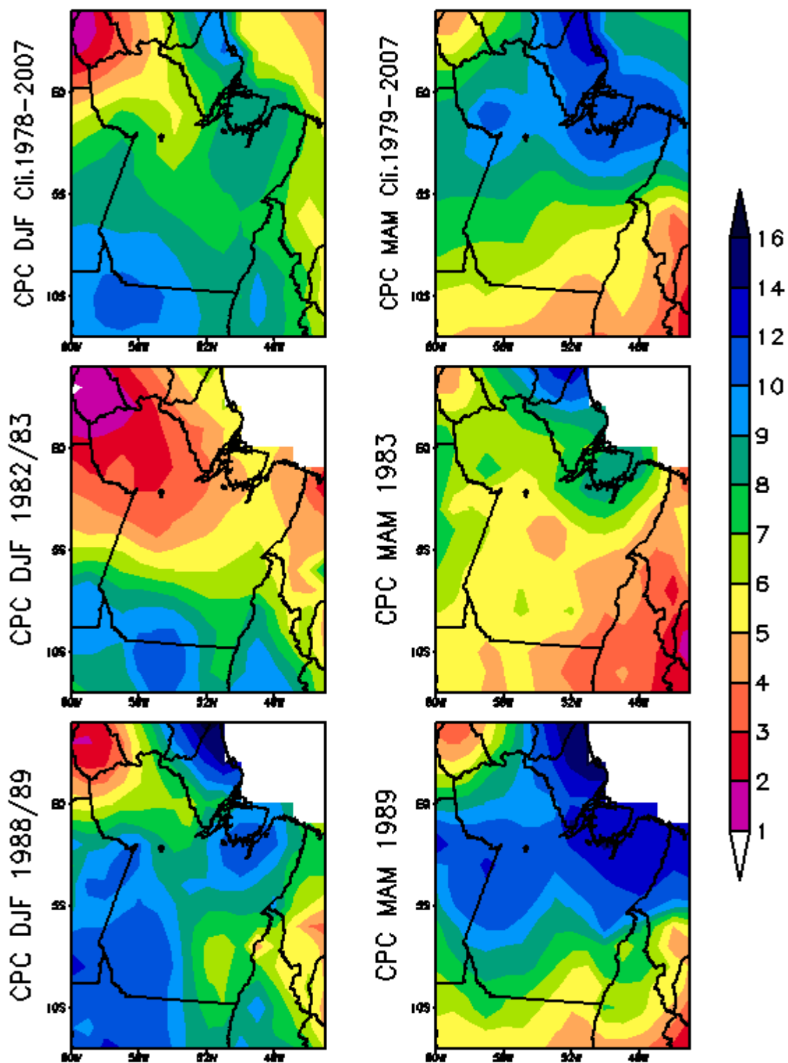
Figura 10. Padrões (distribuição espacial e intensidade) da precipitação (mm/dia) sazonal observada em DJF e MAM correspondentes a climatologia 1979-2008 (mapa superior), 1982/83 (mapa intermediário) e 1988/89 (mapa inferior).
