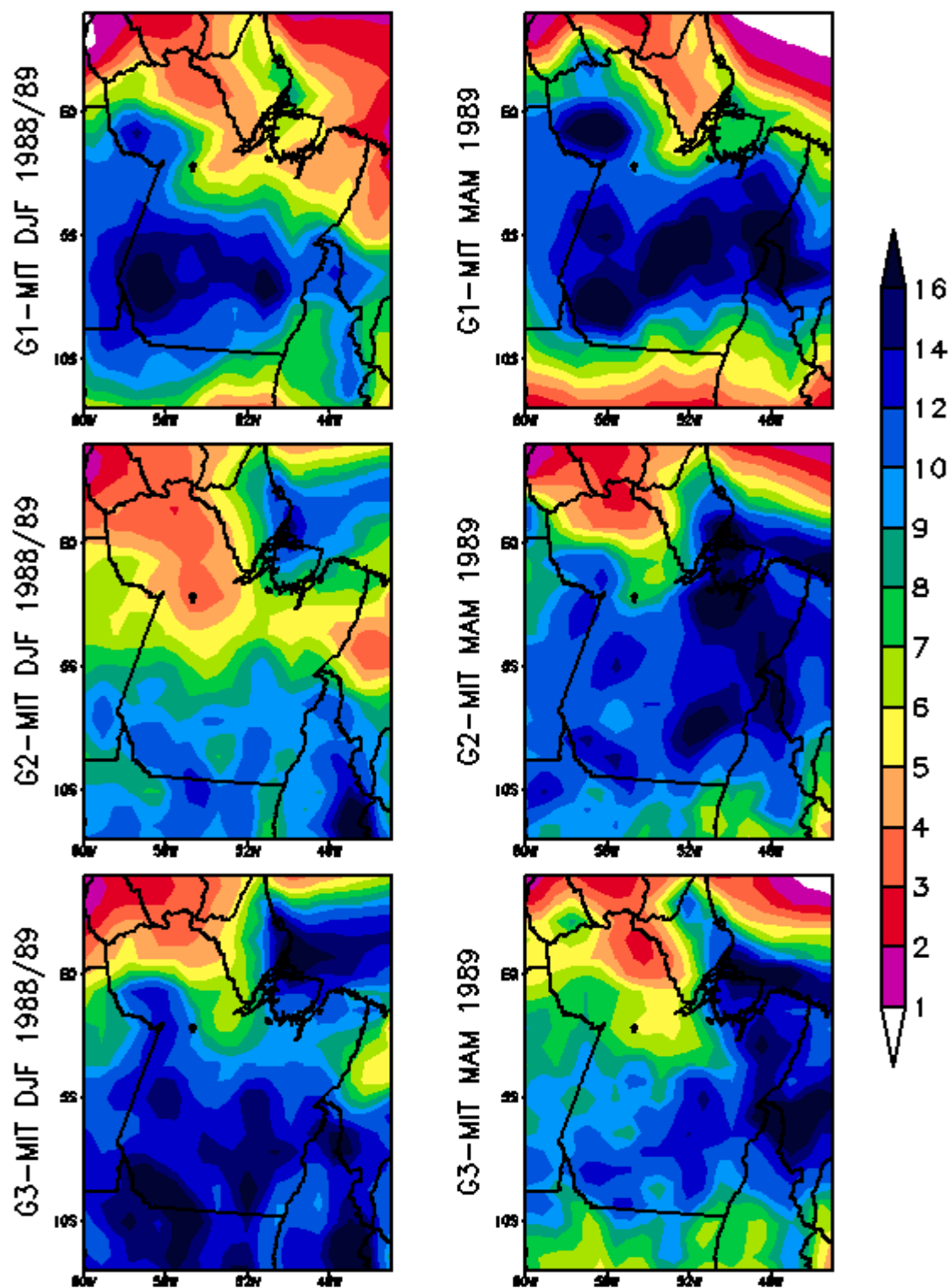
Figura 14. Idem a Figura 13, porém para o esquema convectivo MIT.
