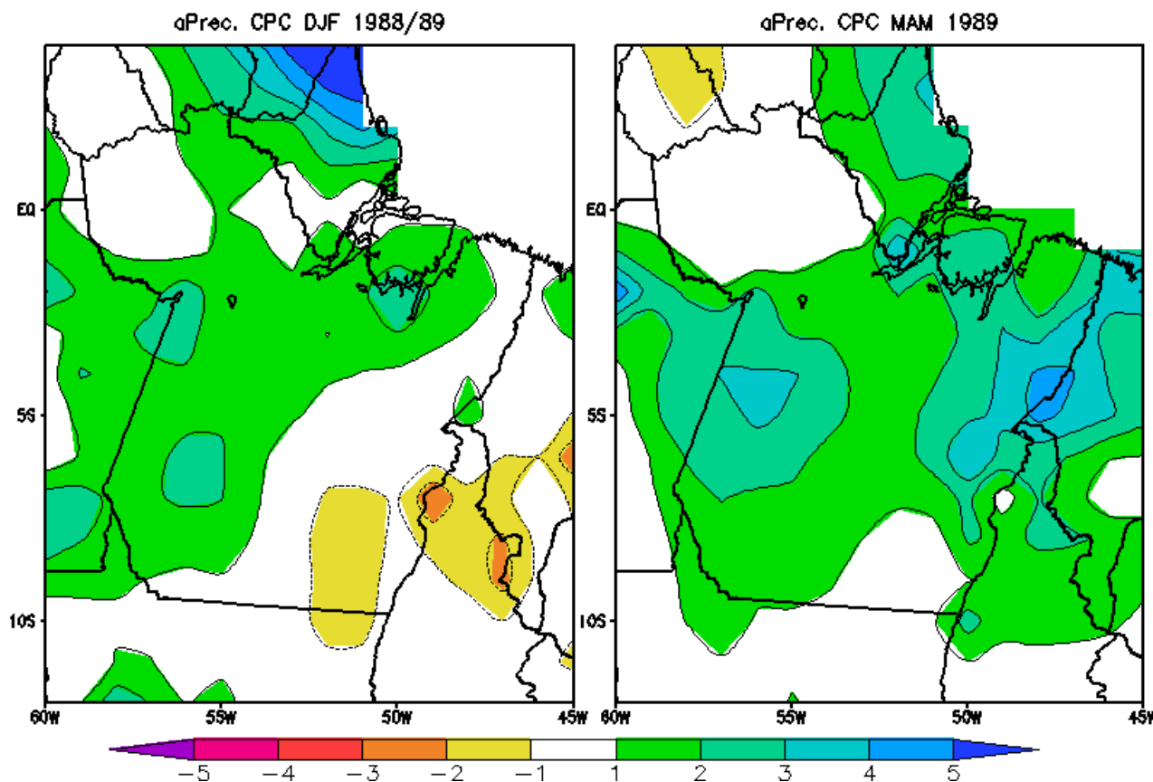
Figura 9. Anomalias de precipitação do CPC observada durante DJF 1988/89 e MAM 1989.
