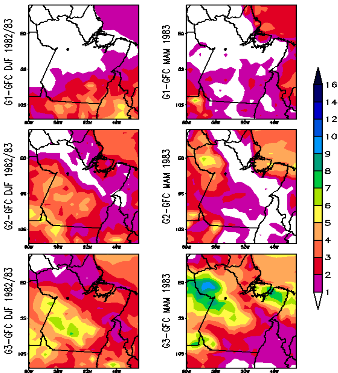
Figura 11. Padrões (distribuição espacial e intensidade) da precipitação (mm/dia) sazonal simulada em DJF 1982/83 e MAM 1983 correspondentes às grades G1 (mapa superior), G2 (mapa intermediário) e G3 (mapa inferior), usando o esquema convectivo GFC.
