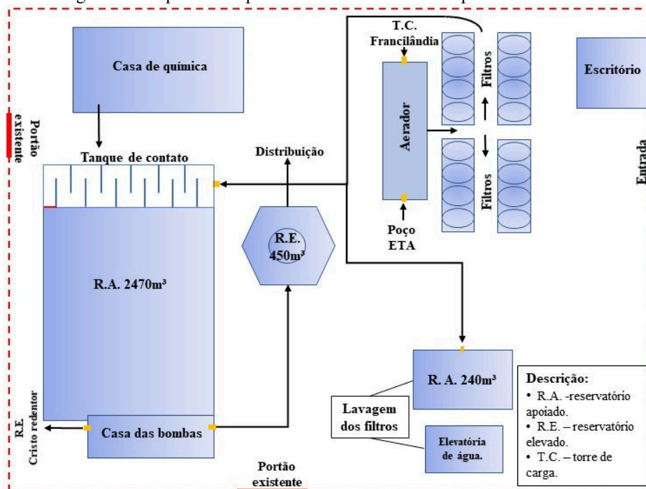
Figura 6 – Sequência de processos da ETA do município de Abaetetuba.
