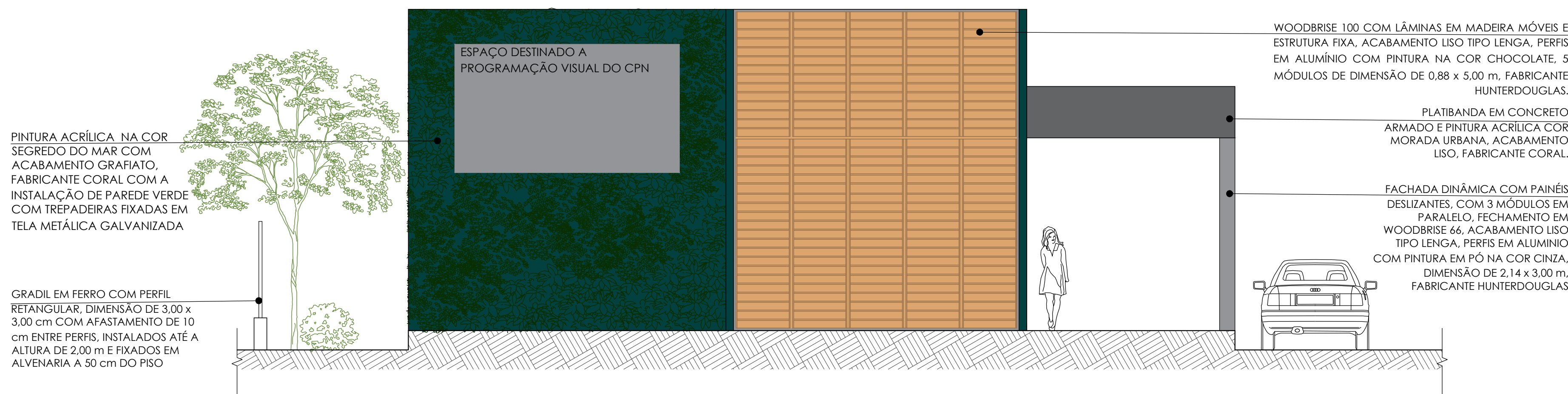
ELEVAÇÃO 01 ESC: 1/50
