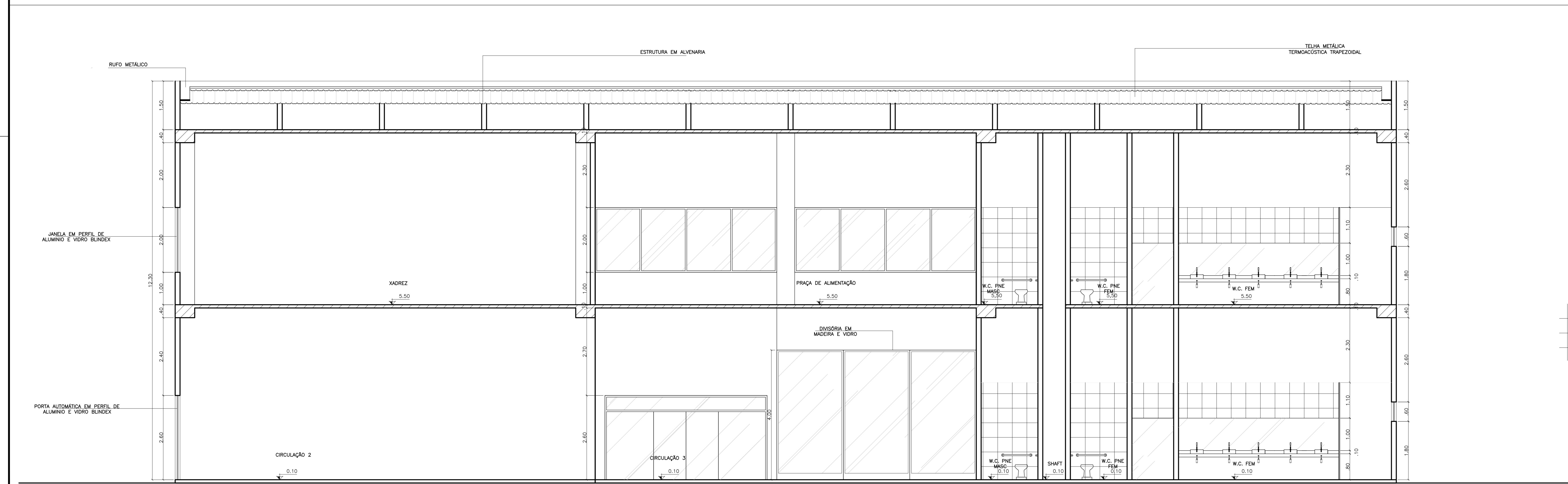
CORTE B esc. 1:50
