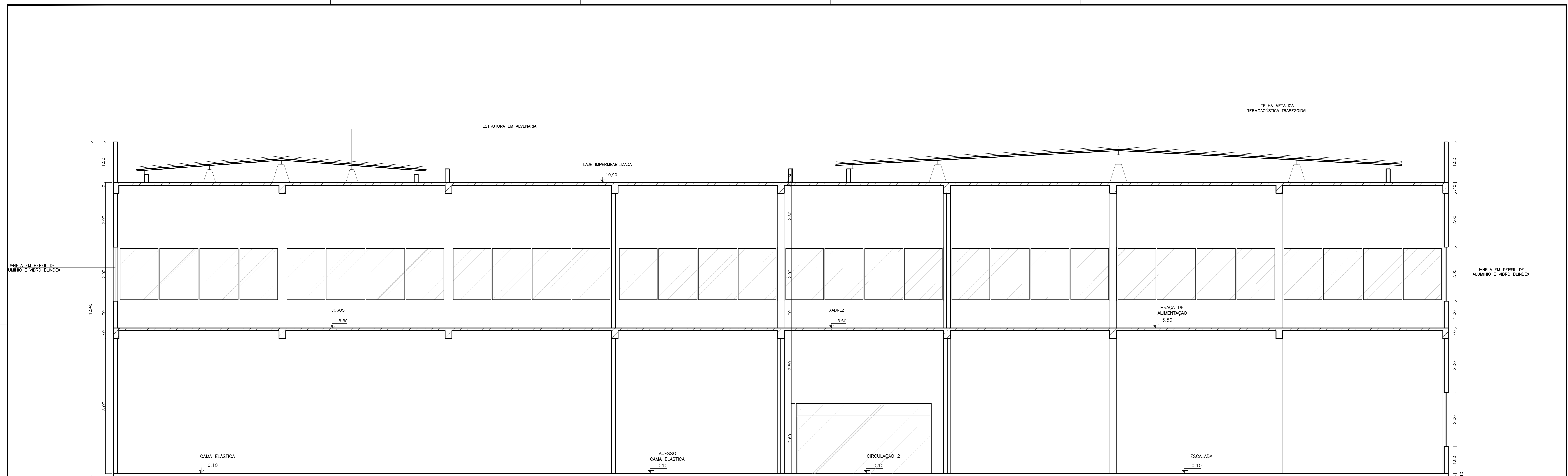
CORTE A esc. 1:50
