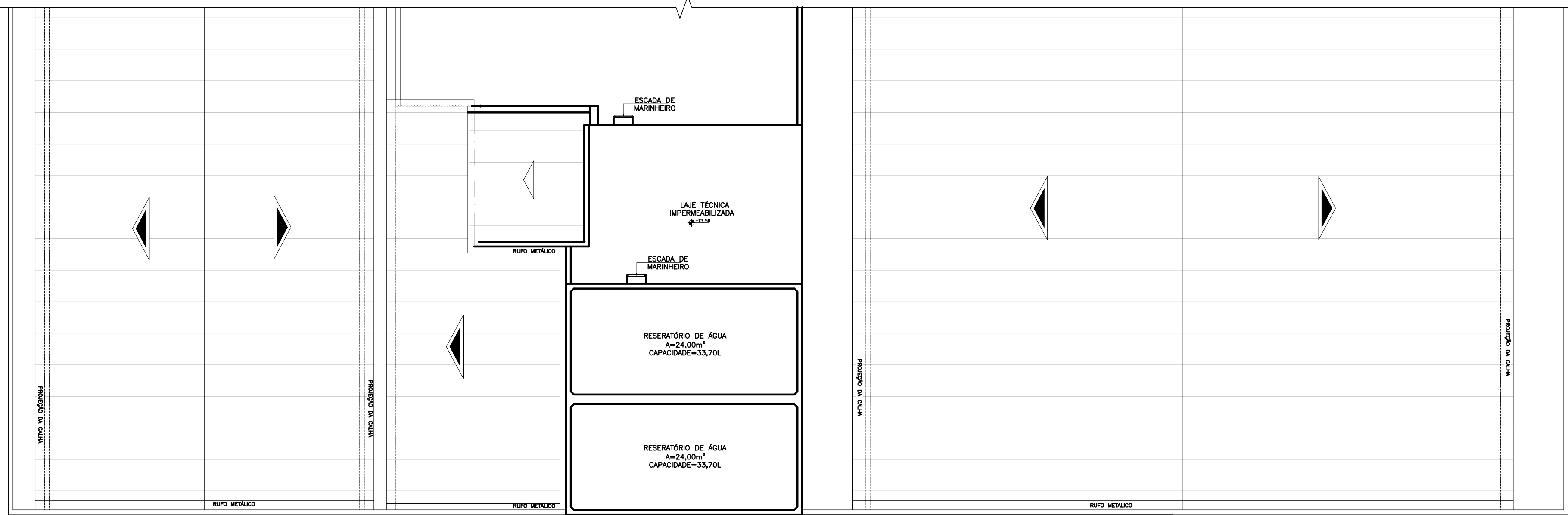
PLANTA BAIXA - COBERTURA esc. 1:100
