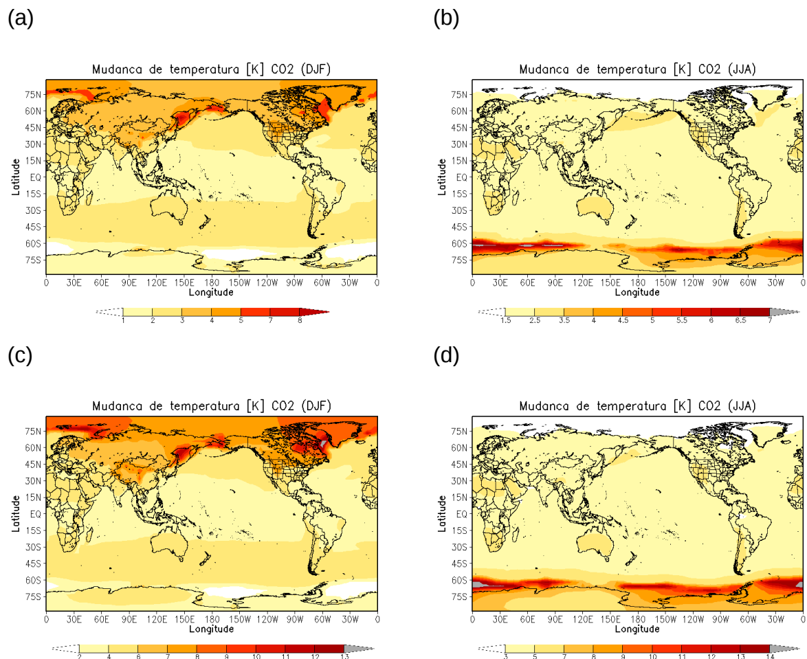
Figura 8 - Simulação do padrão de temperatura obtida com o modelo GREB utilizando a parametrização proposta no trabalho e aumentando em 2 e 4 vezes a concentração de CO 2 : (a) 2x CO 2 Verão, (b) 2x CO 2 Inverno, (c) 4x CO 2 Verão e (d) 4x CO 2 Inverno.
