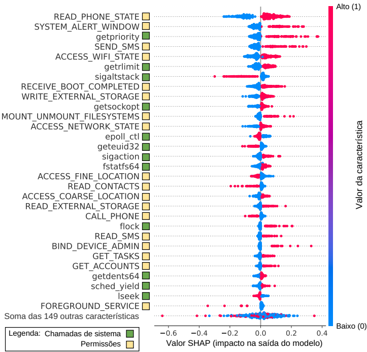
Figura 2. Gráfico SHAP do tipo beeswarm das 30 principais características, em ordem decrescente de acordo com seu impacto na saída do modelo.
