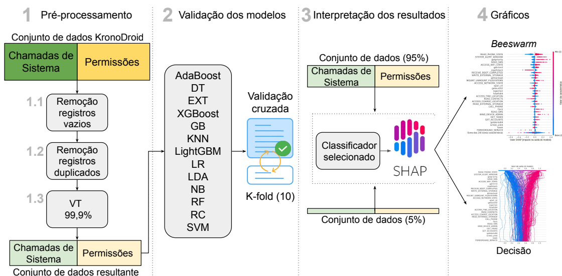
Figura 1. Fluxograma da metodologia na interpretação dos resultados proposta.
