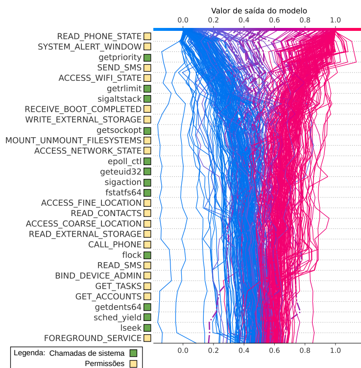
Figura 3. Gráfico SHAP do tipo decisão das 30 principais características, em ordem decrescente de acordo com seu impacto na saída do modelo.
