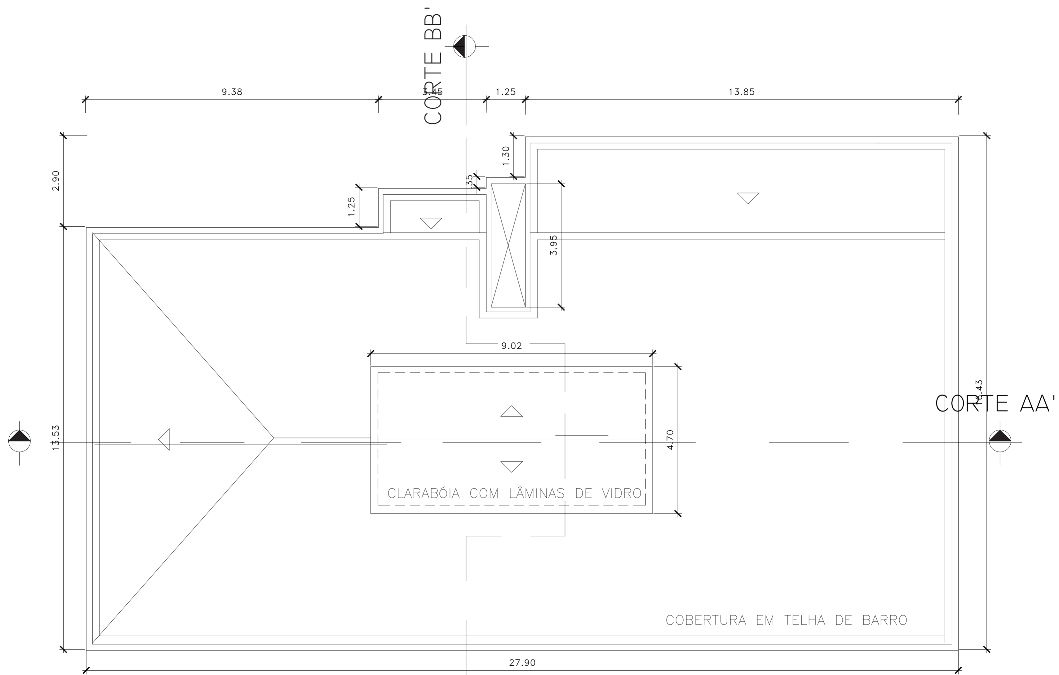
PLANTA DE COBERTURA Esc 1:75
