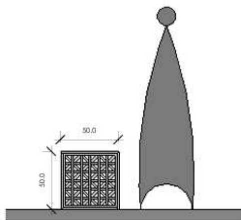
1 ELEVAÇÃO GERAL 1 : 25
