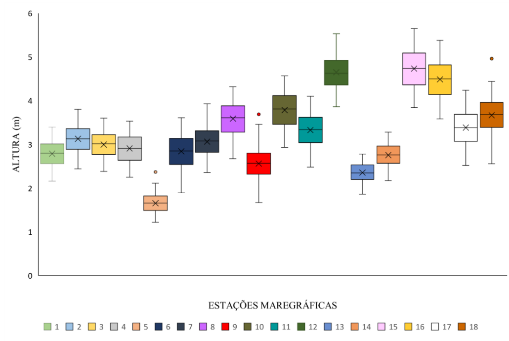
Figura 3 – Boxplot dos dados de preamar para o ano de 2021.
