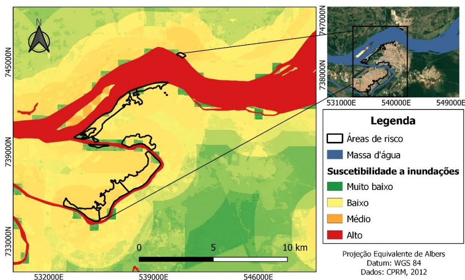
Figura 8 –Inundações na área analisada na parte sul.
