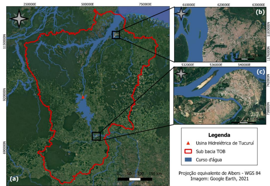
Figura 5- Áreas seleccionadas para validação do ISI
