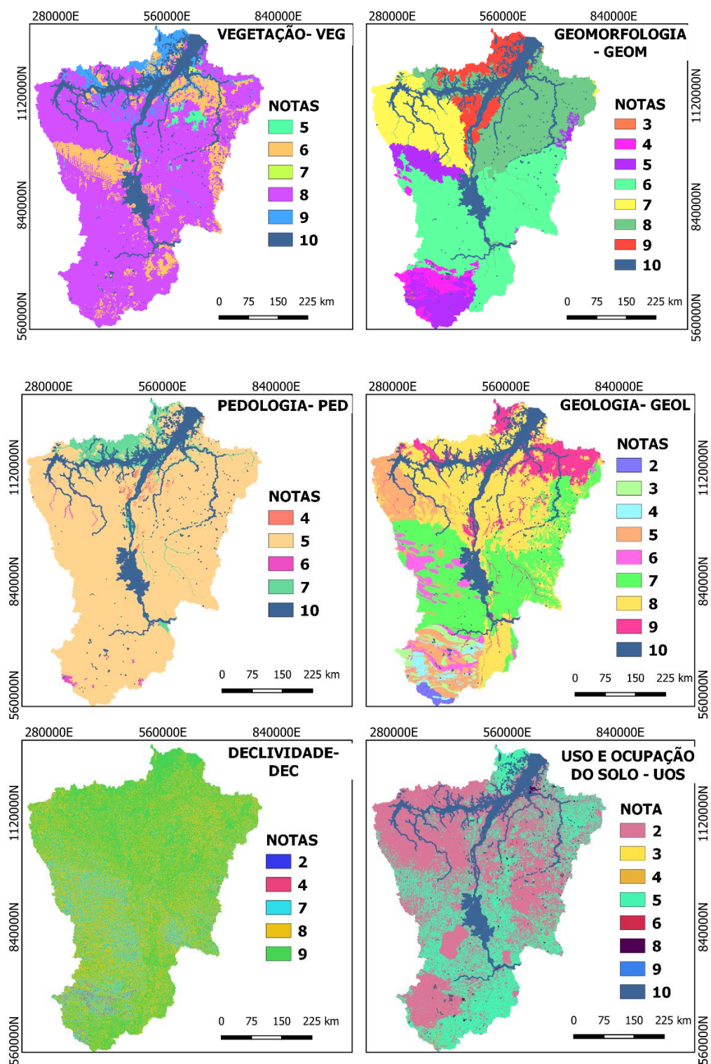
Figura 4- Mapas temáticos dos componentes ambientais.
