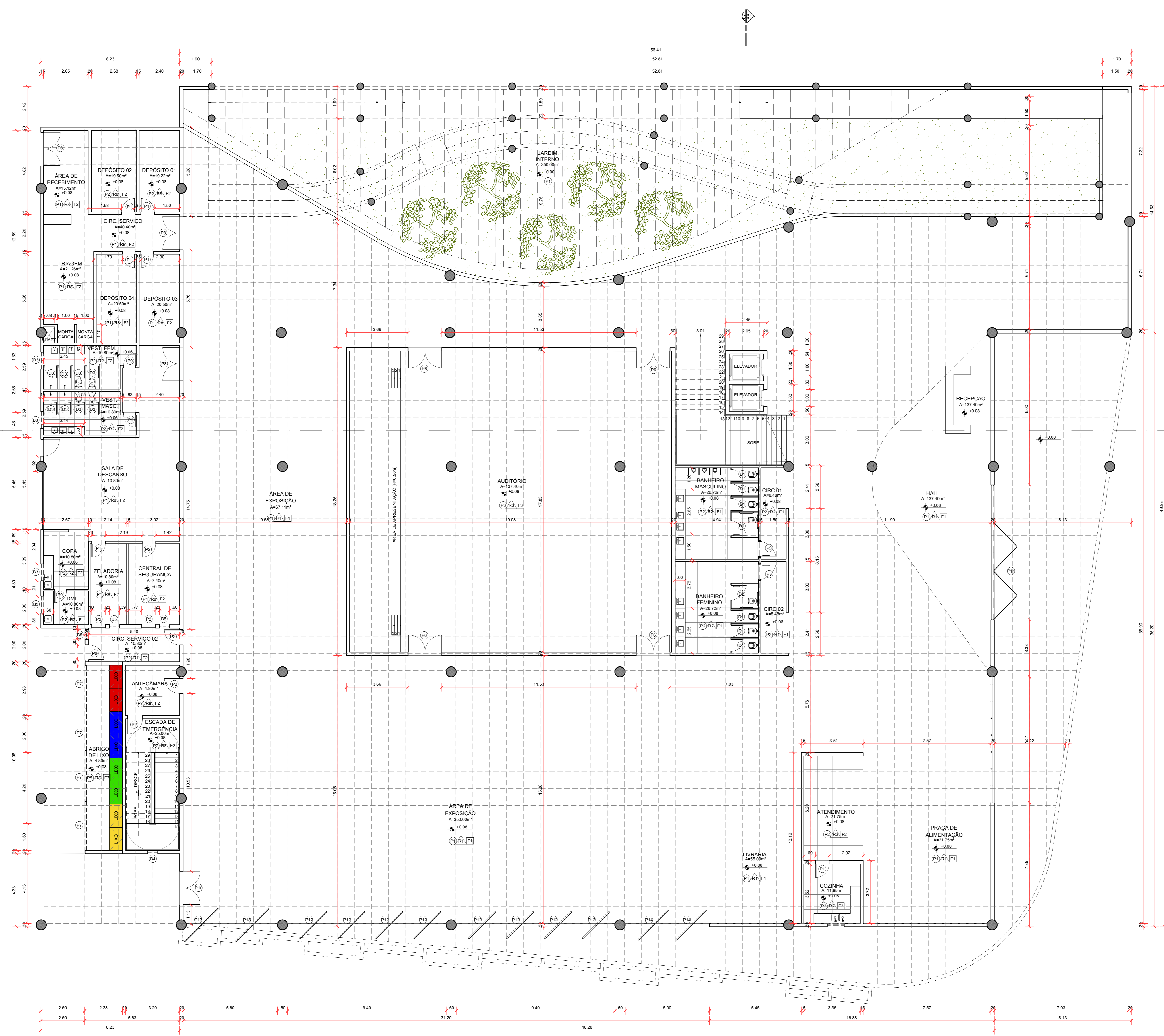
PLANTA BAIXA - PAV. TÉRREO ESC. 1/100
