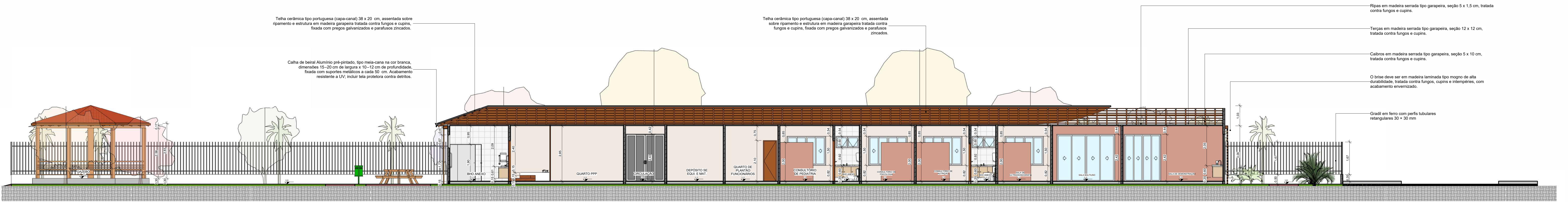
1 CORTE-A 1 : 75
