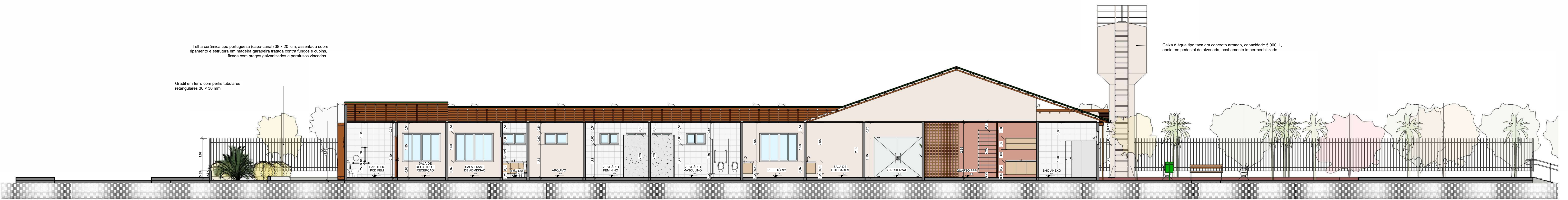
2 CORTE-B 1 : 75
